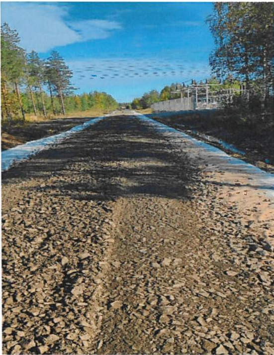
Kuva 5 Suodatin kankaan ja murskeen asennusta
